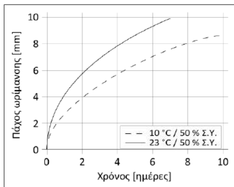
Διάγραμμα 1: Ταχύτητα ωρίμανσης του Sikaflex®-290 DC PRO
