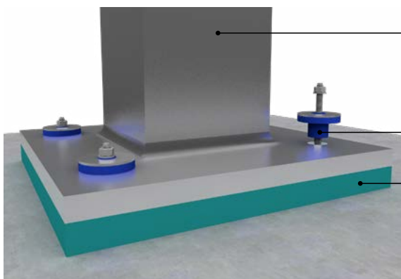
Στήριξη μεταλλικής κατασκευής με Regufoam
