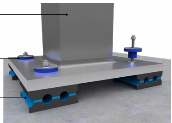
Στήριξη μεταλλικής κατασκευής με Vibro-EP
