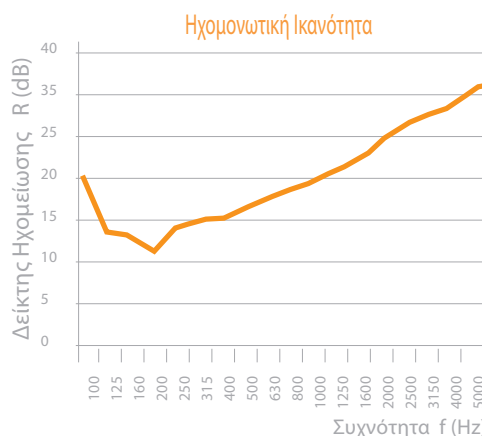
Εργαστηριακή μέτρηση σύμφωνα με ISO 140.3 & ISO 717.1
