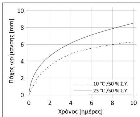
Διάγραμμα 1: Ταχύτητα ωρίμανσης Sikaflex®-552 AT
