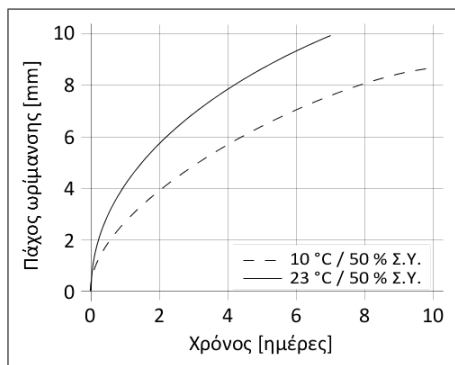
Διάγραμμα 1: Ταχύτητα ωρίμανσης του Sikaflex®-227
